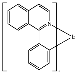
Ir(piq) 3
