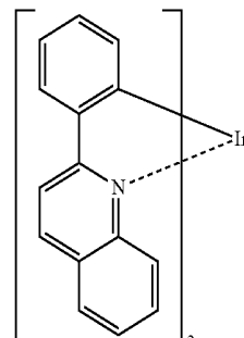
Ir(2-phq) 3
